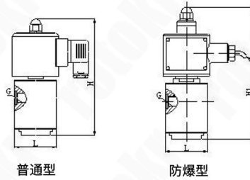
螺纹连接外形尺寸图
